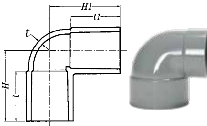
90° L型異徑接頭 90° Reducer Elbow 單位: mm
