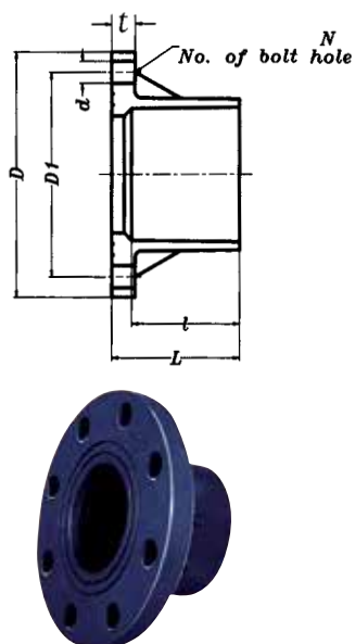
法蘭接頭 Flange
